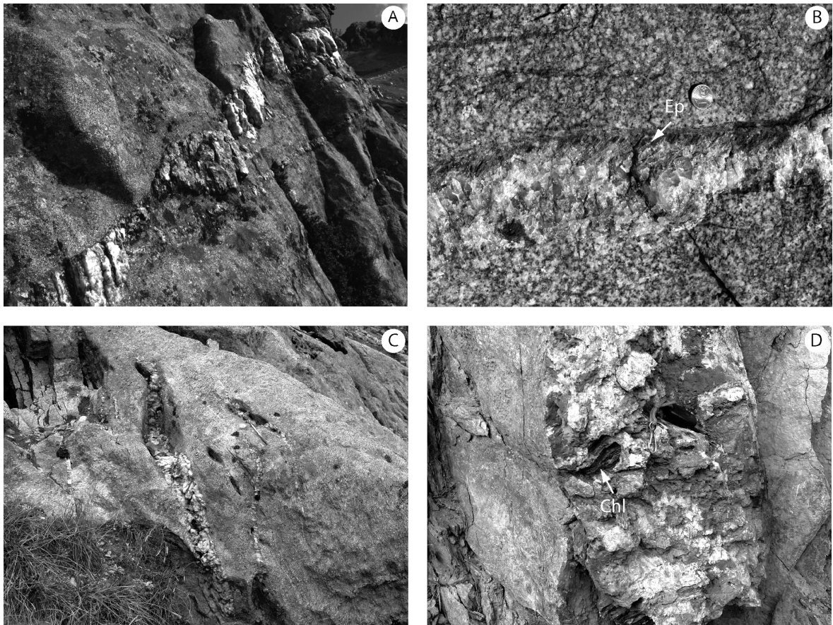
FIG. 4. – Quartz veins. A: Branlay lake (area 4), several flat-lying quartz + epidote veins cross-cut by a later flexuous and oblique veins with large quartz crystals. B: Branlay lake (area 4), detail of a flat-lying quartz + epidote vein. Epidote (Ep) crystallised as sub-vertical fibres. C: Entre-deux-Roches (area 5), en echelon quartz veins. D: Naves road (area 1), vertical vein with chlorite (Chl) and calcite showing flexuous sub-horizontal fibres. FIG. 4. – Veines de quartz. A : lac de Branlay (affleurement 4), plusieurs veines de quartz + épidote de faible pendage sont recoupées par une veine plus tardive, flexueuse, formée de grands cristaux de quartz. B : lac de Branlay (affleurement 4), détail d'une veine de quartz + épidote à faible pendage. L'épidote (Ep) a cristallisé en fibres sub-verticales. C : Entre-deux-Roches (affleurement 5), veines de quartz en échelon. D : route de Naves (affleurement 1), veine de quartz verticale à chlorite (Chl) et calcite montrant des fibres flexueuses sub-horizontales.
