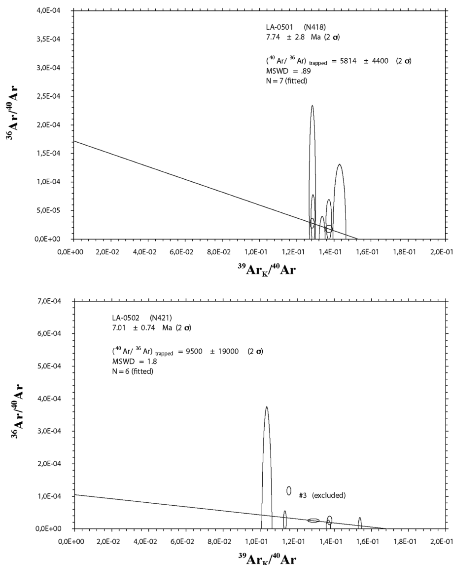
FIG. 8. – Diagrammes isochrones pour l’argon.
