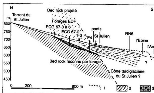
Fig. 6 : Coupe géologique transversale interprétative de la vallée de l'Arc au niveau de Saint Julien. (1) : Cône de déjection récent, (2) : Cône de déjection holocène, (3) : Eroulement rocheux.
