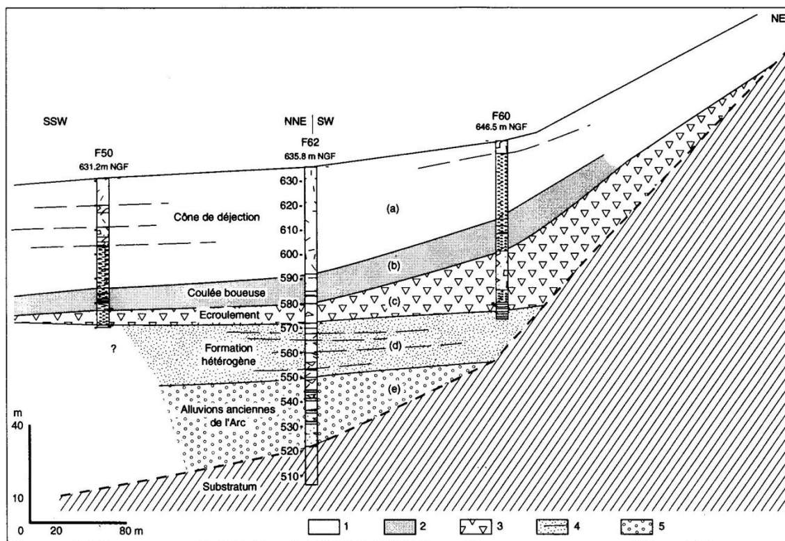
Fig. 5 : Le remplissage torrentiel dans le secteur de Saint Barthélemy (voir localisation sur la figure 2). (1) : Cône de déjection, (2) : Coulées boueuses, (3) : Eroulement, (4) : Formation hétérogène, (5) : Alluvions « anciennes » de l'Arc. Fig. 5 : Torrential filling in the Saint Barthélemy area (see location on figure 2). (1) : Alluvial cone, (2) : Mud flow, (3) : Side fall, (4) : Heterogeneous formation, (5) : Old alluvial deposits of the Arc river.
