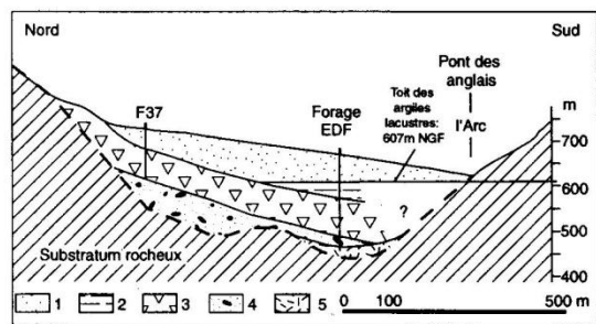
Fig. 9 : Coupe géologique transversale de la vallée au niveau du forage EDF profond du Claret. (1) : Cône holocène à récent du Claret, (2) : Argiles lacustres, (3) : Ecoulement de versant, (4) : Cône ancien du Claret, (5) : Moraine de fond (?).
