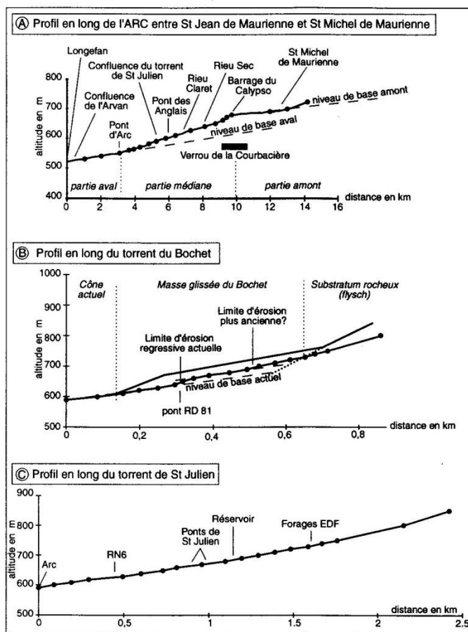
Fig. 3 : Analyse des profils en long des torrents. Fig. 3 : Analysis of the torrent lengthways section.
