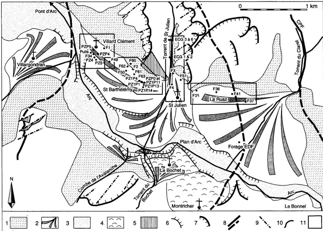
Fig. 2 : Cadre morphologique de la région de Saint Julien Montdenis et localisation des sondages. (1) : Eboulis, (2) : Cône de déjection, (3) : Alluvions récentes de l'Arc, (4) : Glissement de versant, (5) : Facette triangulaire, (6) : Limite d'ablation des cônes anciens, (7) : Niche d'arrachement, (8) : Contact tectonique (a) observé, (b) masqué, (9) : Failles déduites de la morphologie, (10) : Cours d'eau, (11) : Substratum rocheux indifférencié.
