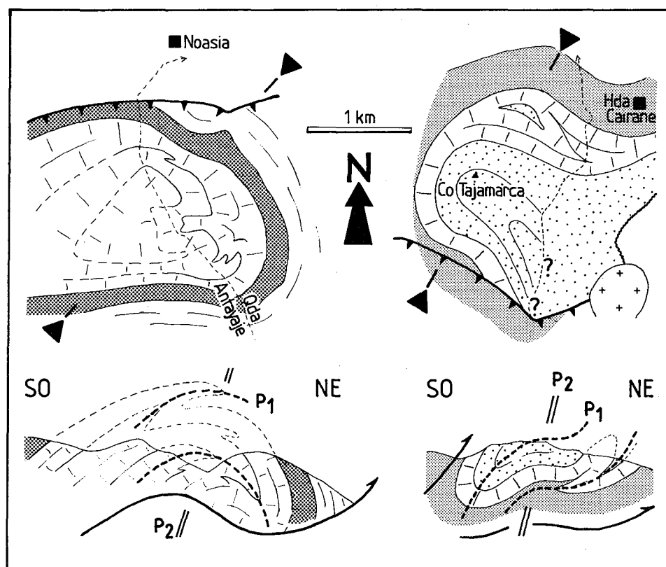
Fig. 6 - Mapas (arriba) y cortes (abajo) simplificados e interpretativos de la estructura polifásica de la quebrada Antayaje, y del Cerro Tajamarca (para su ubicación, ver en la Fig. 4). Misma leyenda que en la figura 4. P1 y P2: Planos axiales de los pliegues de fase 1 y 2 respectivamente.
