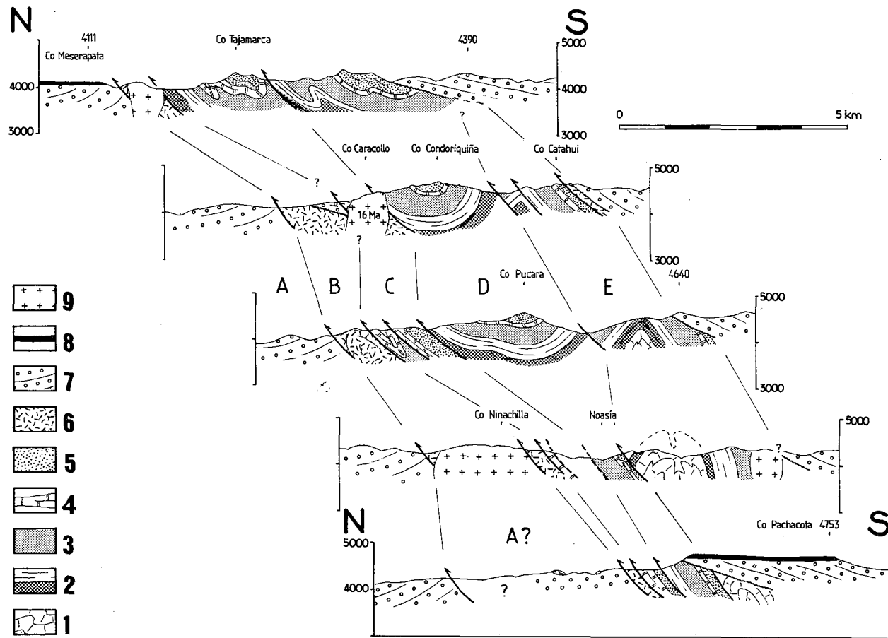
Fig. 5 - Cortes geológicos en la zona de Mañazo. Mismas leyendas que en la figura 4. Las letras A a E se refieren a las unidades tectónicas descritas en el texto. De arriba hasta abajo, los perfiles se enlazan del Este al Oeste (ver en la Fig. 4).
