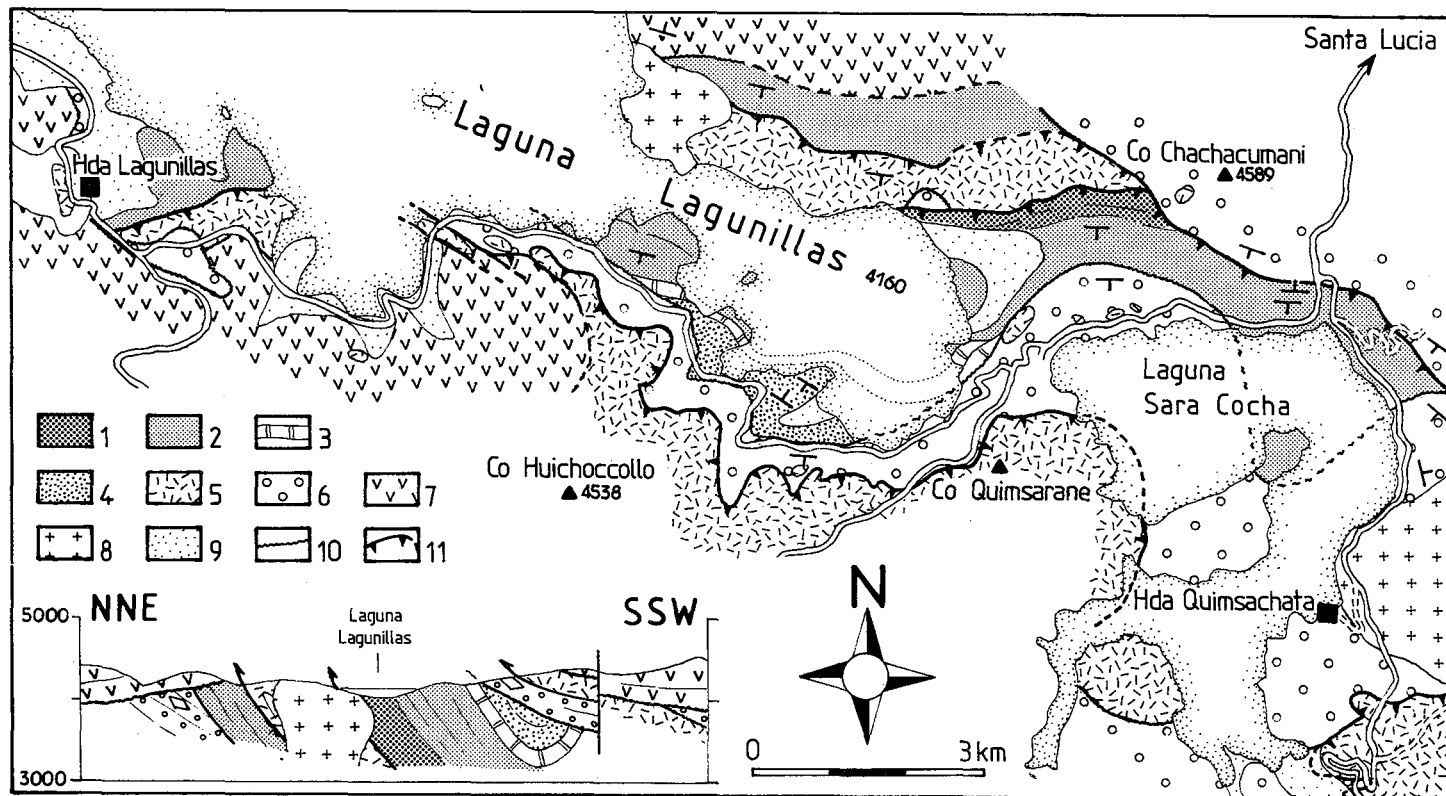
Fig. 7 - Mapa geológico de la zona de la Laguna Lagunillas, y corte simplificado. El corte pasa aproximadamente por el Cerro Huichoccollo. 1: Unidad lutácea del Grupo Lagunillas (Calloviano - Oxfordiano); 2: Unidad cuarcítica del Grupo Lagunillas (Oxfordiano superior ? y Kimmeridgiano); 3: Unidad calcárea superior del Grupo Lagunillas (Tithoniano); 4: Formaciones Hualhuani y Murco (Valanginiano - Aptiano); 5: Formaciones Huambo y Arcurquina (Aptiano superior ? - Turoniano); 6: Grupo Puno (Oligoceno inferior a medio) localmente con olistolitos; 7: Grupo Tacaza (Oligoceno superior - Mioceno inferior); 8: Cuerpos intrusivos; 9: Depósitos cuaternarios; 10: Discordancias; 11: Sobre - escurrimientos.
