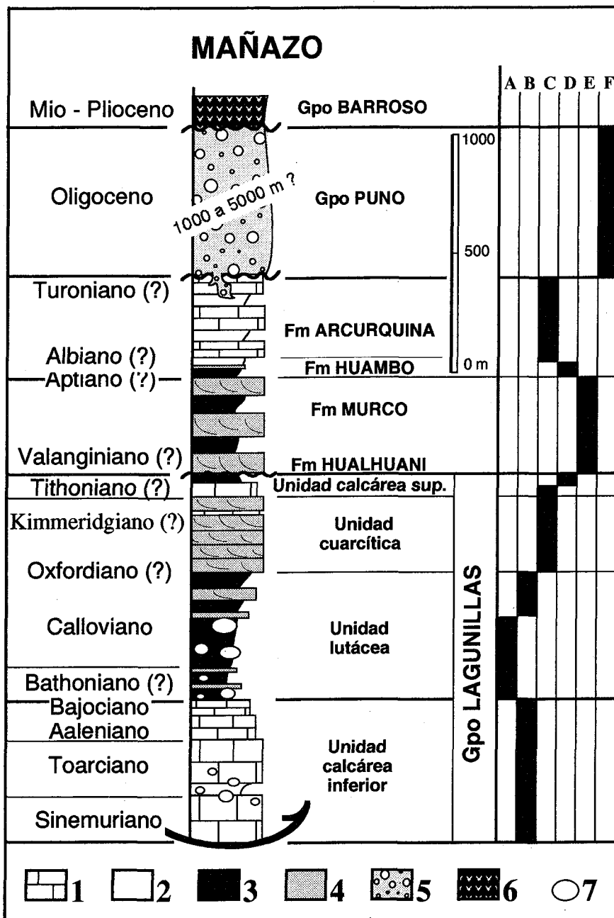
Fig. 2 - Columna sintética de la serie de Mañazo-Laguna Lagunillas. Litología: 1: Calizas; 2: Margas; 3: Lutitas; 4: Areniscas; 5: Conglomerados; 6: Rocas volcánicas; 7: Olistolitos. Ambientes de depósito: A: Pelágico; B: Hemi-pelágico; C: Plataforma; D: Costero o intertidal; E: Fluvio-deltaico; F: Cono aluvial continental.
