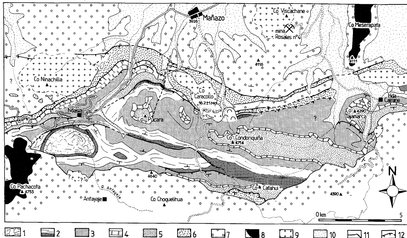
Fig. 4 - Mapa geológico de la zona de Mañazo. 1: Unidad calcárea inferior del Grupo Lagunillas (Sinemuriano superior - Bajociano); 2: Unidad lutácea del Grupo Lagunillas (Bathoniano: abajo y Calloviano - Oxfordiano: arriba); 3: Unidad cuarcítica del Grupo Lagunillas (Oxfordiano superior? y Kimmeridgiano); 4: Unidad calcárea superior del Grupo Lagunillas (Tithoniano); 5: Formaciones Hualhuani y Murco (Valanginiano - Aptiano); 6: Formaciones Huambo y Arcurquina (Aptiano superior? - Turoniano); 7: Grupo Puno (Oligoceno inferior a medio) (Grupo Maure, Mioceno medio a superior al oeste, según Klinck et al. , 1986); 8: Grupo Barroso (Mioceno superior - Plioceno inferior); 9: Cuerpos intrusivos; 10: Depósitos cuaternarios; 11: Discordancias; 12: Sobre-escurrimientos.
