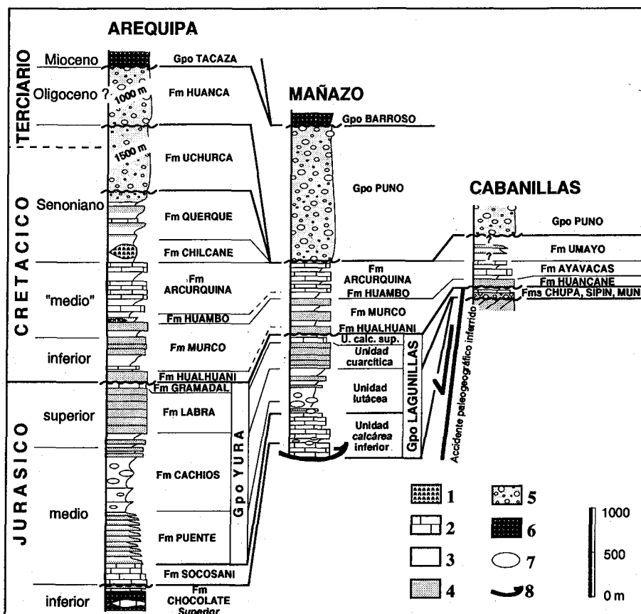
Fig. 3 - Correlaciones de la serie Mañazo con las áreas de Arequipa (Cuenca de Arequipa) y de Cabanillas (eje de Santa Lucía o Cusco-Puno).
