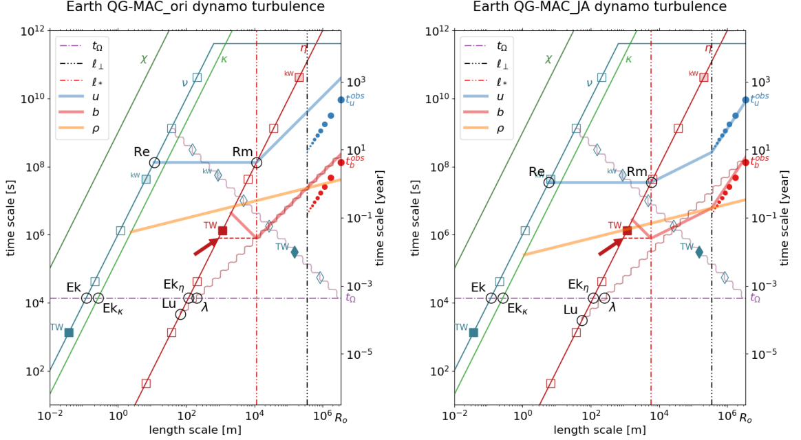
(a) Simple QG-MAC balance scenario.
