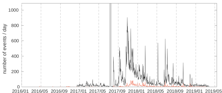
Figure 2 - Nombre d'événements sismiques détectés par SISMalp (rouge) et suite à l'application des méthodes de délocalisation et de détection fine. Au plus fort de la crise, plus de 800 événements par jour ont été détectés. (D'après Janex, 2019)
