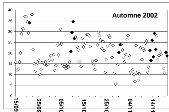
FIG. 1.12 – Eau Précipitable ( \text{kg/m}^2 ) estimée à partir du radiosondage de Nîmes du 15 septembre au 20 novembre 2002. Les journées à plus de 100 mm de précipitation listées dans le tableau 1.1 sont noircies. (source : Météo-France)
