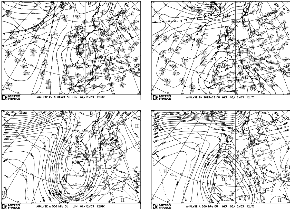
FIG. 1.9 – Analyse des 1 er et 3 décembre 2003 à 12 UTC en surface (haut) et à 500 hPa (bas). Au pointage des observations sont superposés les géopotentiels (trait plein) et la température (trait tiret) à 500 hPa et la pression au niveau de la mer (trait plein) issus de l'analyse ARPEGE. (source : Météo-France)
